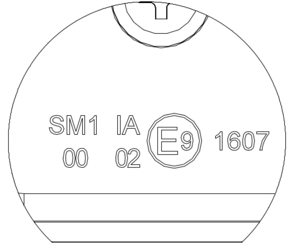
SZCZEGÓŁ A SKALA 5 : 1
